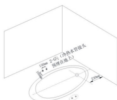
落地式龙头(二)
