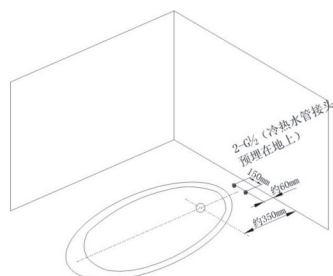
落地式龙头(一)
